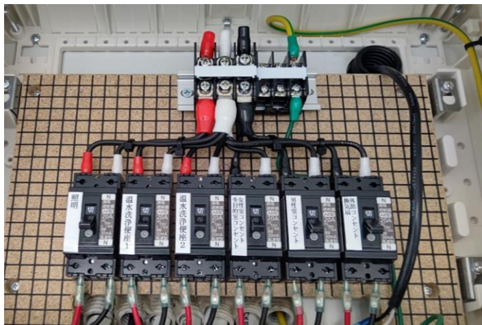
ブレーカー20A×6
